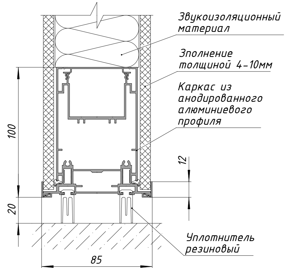
Узел примыкания к полу
